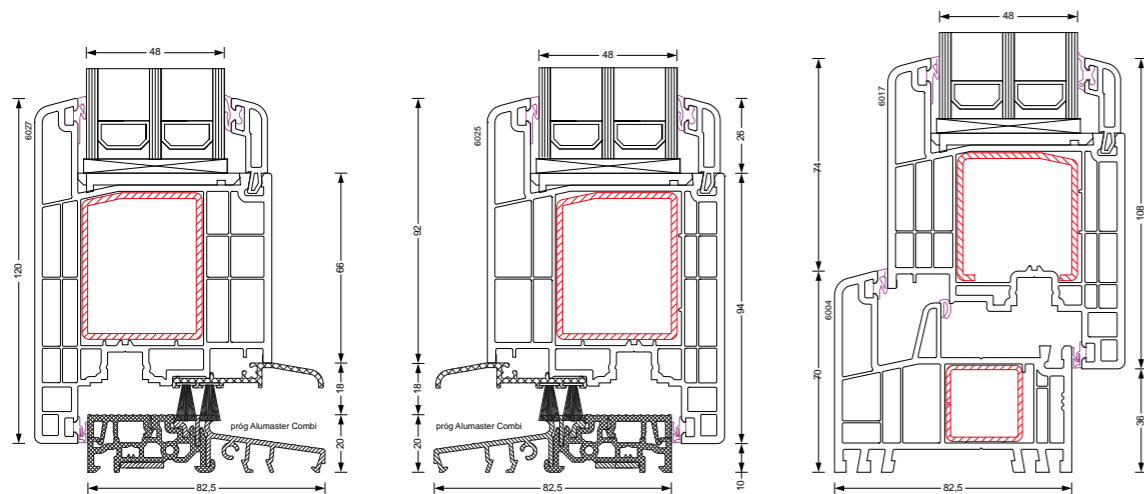
DRZWI OTWIERANE NA ZEWNĄTRZ
